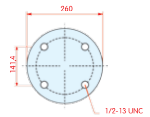
onderaanzicht
