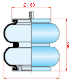
zijaanzicht
