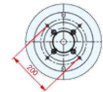
onderaanzicht
