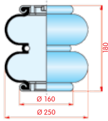
zijaanzicht
