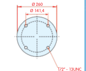
onderaanzicht
