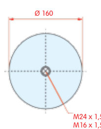
bovenaanzicht
