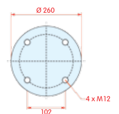
onderaanzicht
