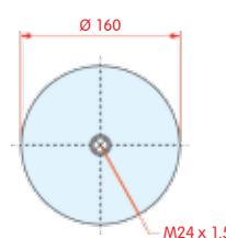
bovenaanzicht
