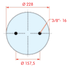
onderaanzicht
