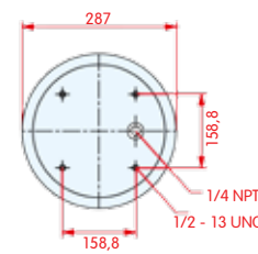
bovenaanzicht
