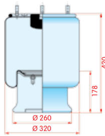
zijaanzicht
