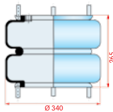
zijaanzicht
