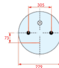
bovenaanzicht
