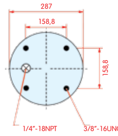
bovenaanzicht
