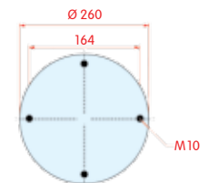
onderaanzicht
