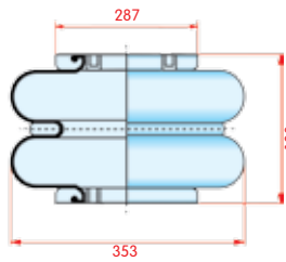
zijaanzicht
