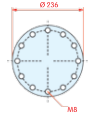
onderaanzicht
