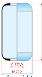
zijaanzicht
