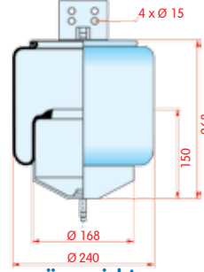
zijaanzicht
