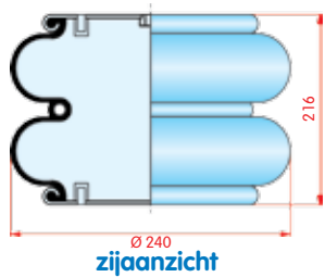
zijaanzicht
