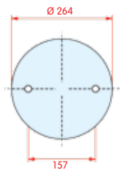
onderaanzicht
