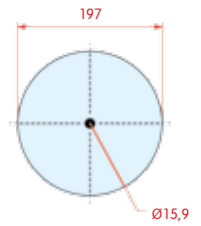
onderaanzicht
