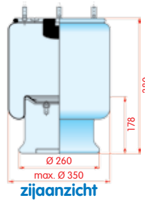
zijaanzicht
