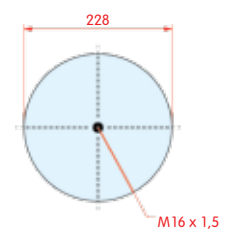
onderaanzicht
