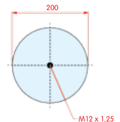
onderaanzicht
