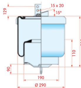
zijaanzicht
