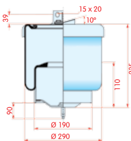
zijaanzicht
