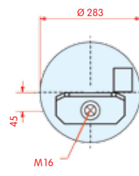
bovenaanzicht
