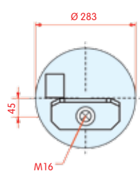
bovenaanzicht
