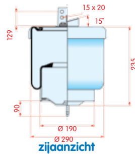
zijaanzicht
