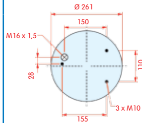
bovenaanzicht
