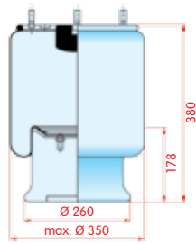
zijaanzicht
