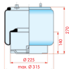
zijaanzicht
