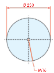
onderaanzicht
