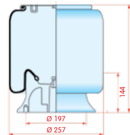
zijaanzicht
