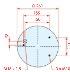
bovenaanzicht
