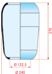
zijaanzicht
