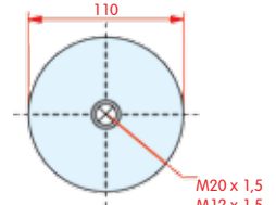
onderaanzicht
