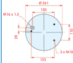
bovenaanzicht
