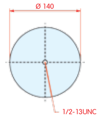
onderaanzicht
