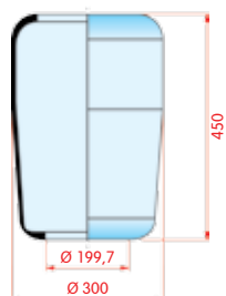
zijaanzicht
