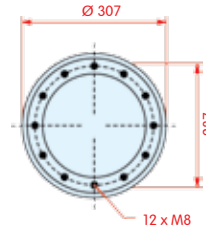
bovenaanzicht
