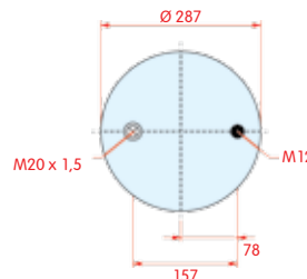
bovenaanzicht
