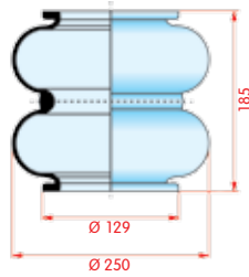
zijaanzicht
