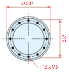
onderaanzicht
