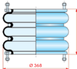
zijaanzicht
