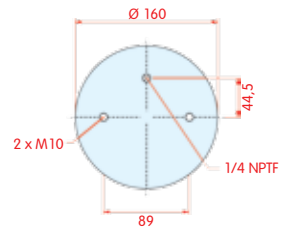
bovenaanzicht
