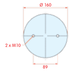
onderaanzicht
