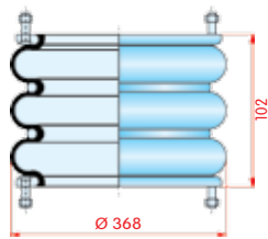
zijaanzicht
