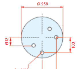
onderaanzicht
