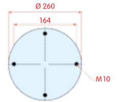
onderaanzicht
