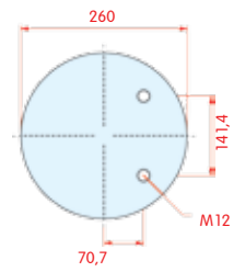
onderaanzicht
