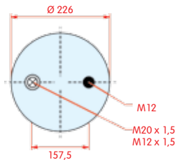
bovenaanzicht
