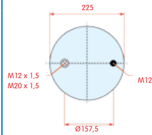
bovenaanzicht
