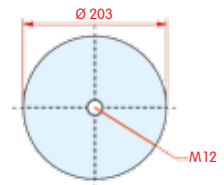
onderaanzicht
