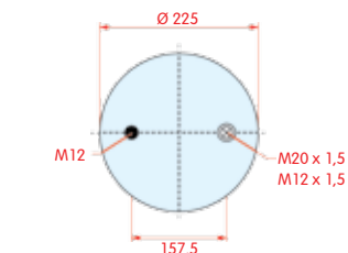
bovenaanzicht
