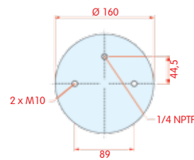
bovenaanzicht
