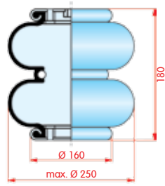
zijaanzicht
