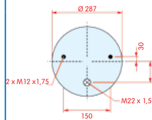
bovenaanzicht
