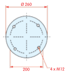
onderaanzicht
