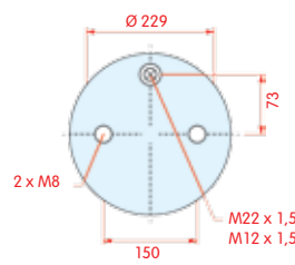
bovenaanzicht
