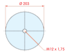
onderaanzicht
