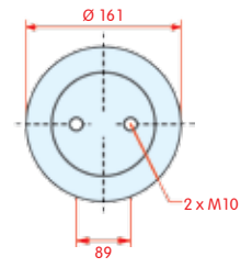
onderaanzicht
