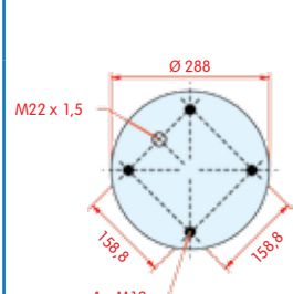
bovenaanzicht
