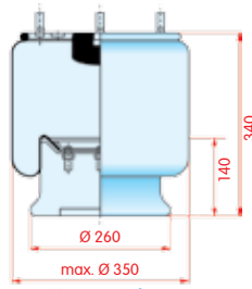
zijaanzicht
