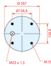
bovenaanzicht
