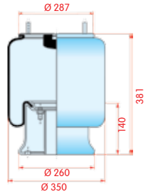
zijaanzicht
