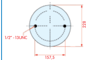
onderaanzicht
