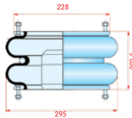
zijaanzicht
