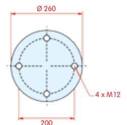
onderaanzicht
