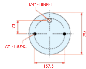
bovenaanzicht
