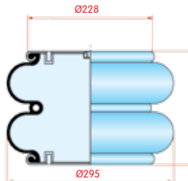
zijaanzicht
