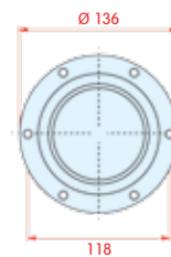
bovenaanzicht
