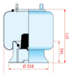
zijaanzicht
