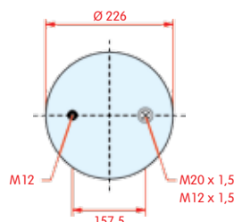
bovenaanzicht
