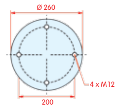
onderaanzicht
