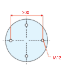
onderaanzicht
