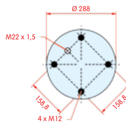
bovenaanzicht
