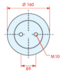
onderaanzicht
