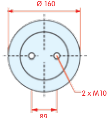
onderaanzicht
