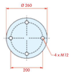
onderaanzicht
