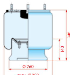
zijaanzicht
