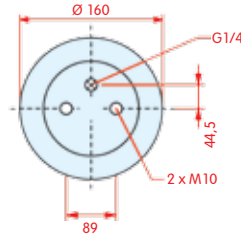
bovenaanzicht
