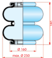
zijaanzicht
