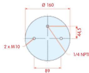
bovenaanzicht
