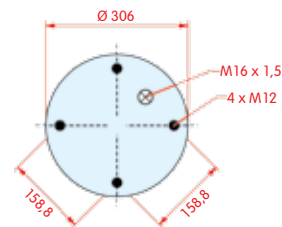
bovenaanzicht
