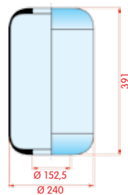
zijaanzicht
