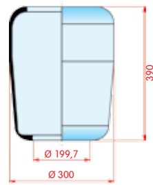
zijaanzicht
