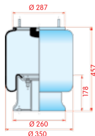
zijaanzicht
