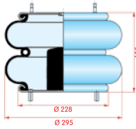
zijaanzicht
