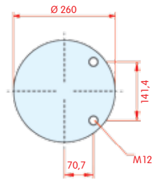
onderaanzicht
