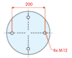
onderaanzicht
