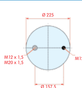
bovenaanzicht
