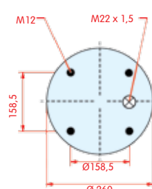
bovenaanzicht
