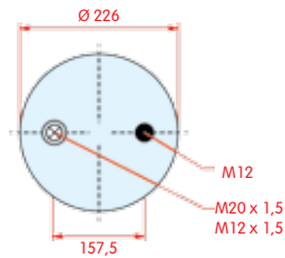
bovenaanzicht
