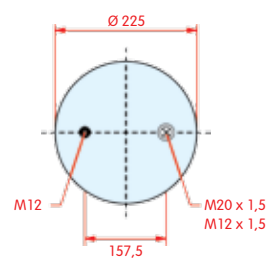
bovenaanzicht
