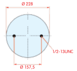
onderaanzicht
