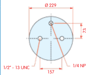
bovenaanzicht
