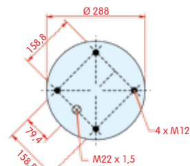
bovenaanzicht
