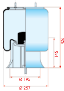
zijaanzicht
