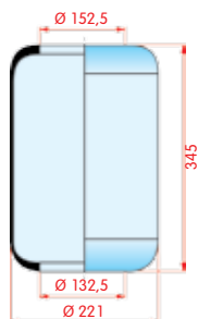
zijaanzicht
