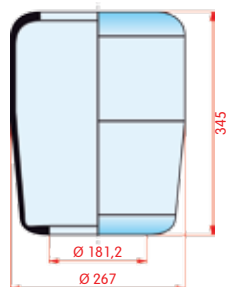
zijaanzicht
