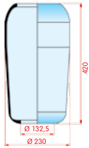
zijaanzicht
