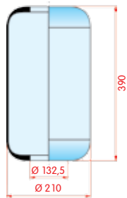
zijaanzicht
