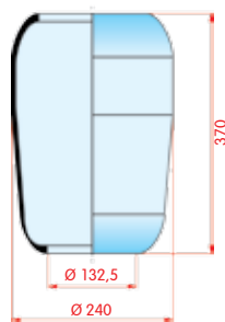
zijaanzicht
