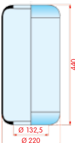
zijaanzicht
