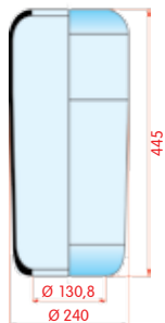
zijaanzicht
