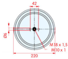
bovenaanzicht
