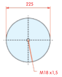
onderaanzicht
