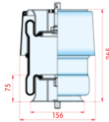
zijaanzicht
