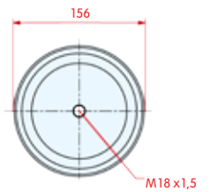
onderaanzicht
