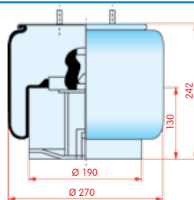
zijaanzicht
