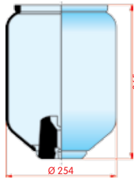
zijaanzicht
