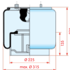
zijaanzicht
