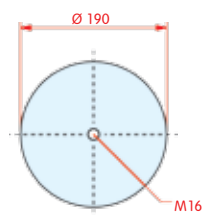
onderaanzicht
