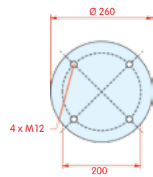
onderaanzicht
