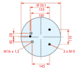
bovenaanzicht
