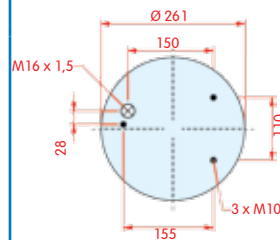
bovenaanzicht
