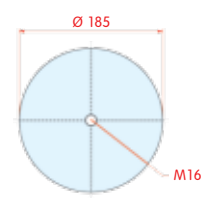
onderaanzicht
