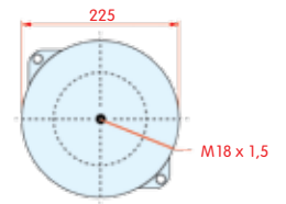
onderaanzicht
