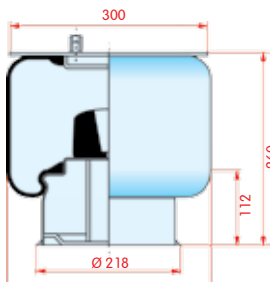
zijaanzicht
